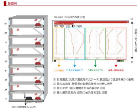
構造ヘルスマモニタリング 設置イメージ
