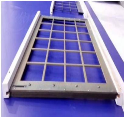
ソーラーパネル用 C/C コンポジット製サセプター。 熱による歪みが少ないのが特徴
