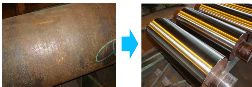
肉盛溶接によるロール(ローラー)の再生補修例
