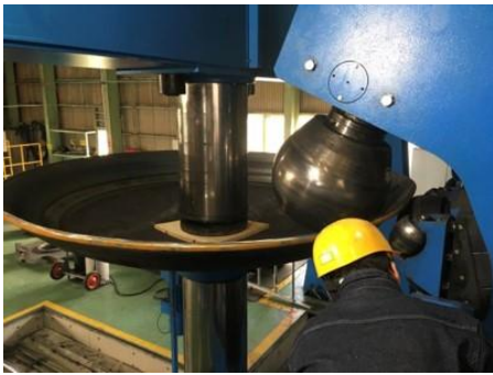
スピニングマシン による鏡板製作
